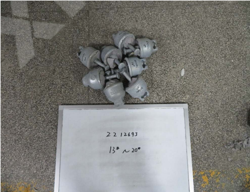
残留机械强度试验状况照片1
